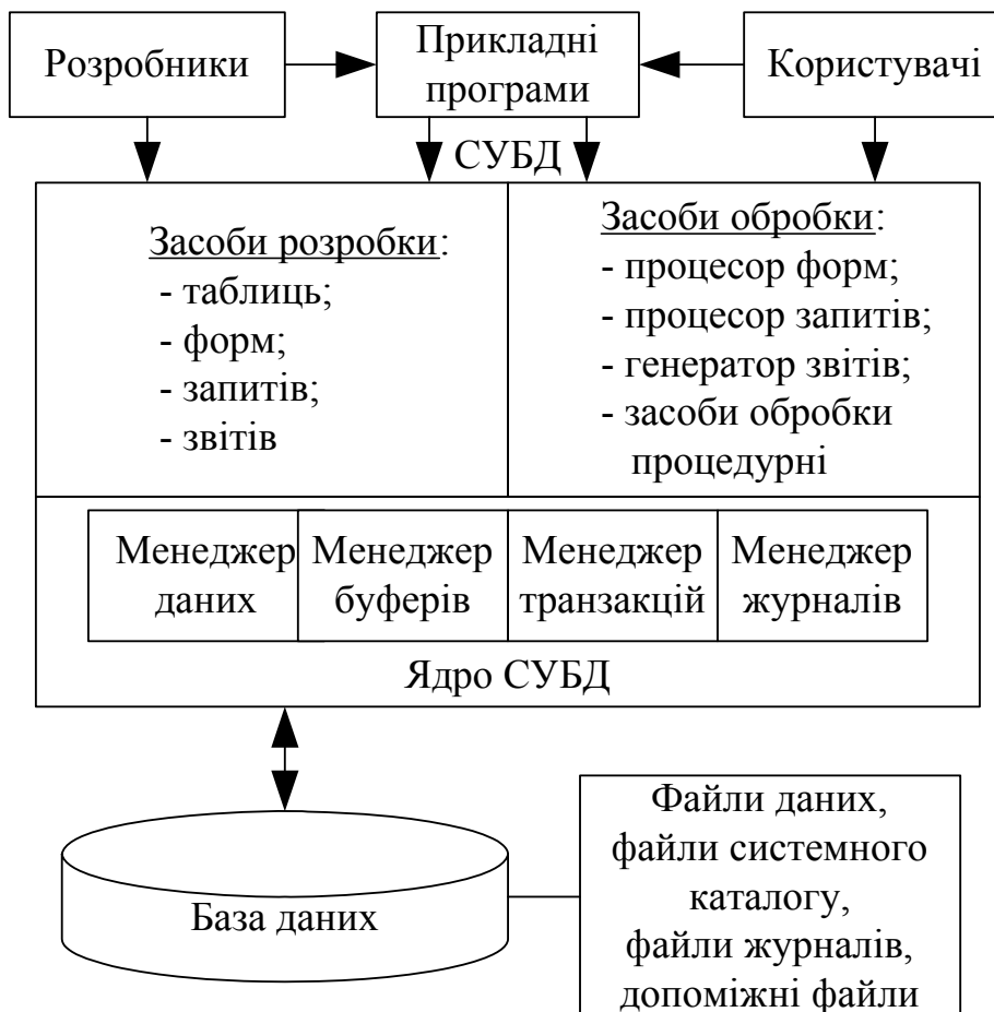
Рис. 1.4. Компоненти системи бази даних
