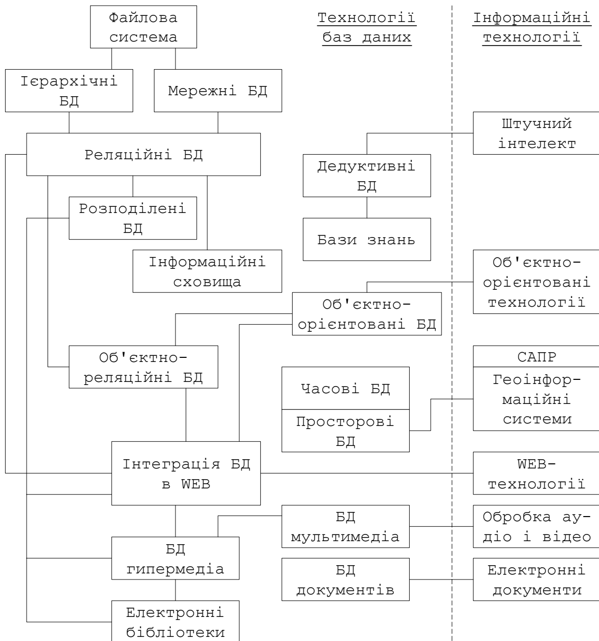
Рис. 1.2. Етапи розвитку баз даних
