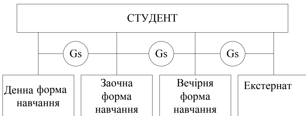
Рис. 5.15. Діаграма зв'язку суперкласу з підкласом з обов'язковою участю
