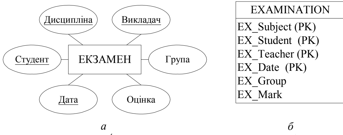
Рис. 6.24. Перетворення сутності Екзамен (а) у відношення Examination (б)
