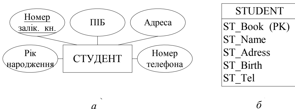
Рис. 6.9. Перетворення сутності Студент (а) у відношення Student (б)
