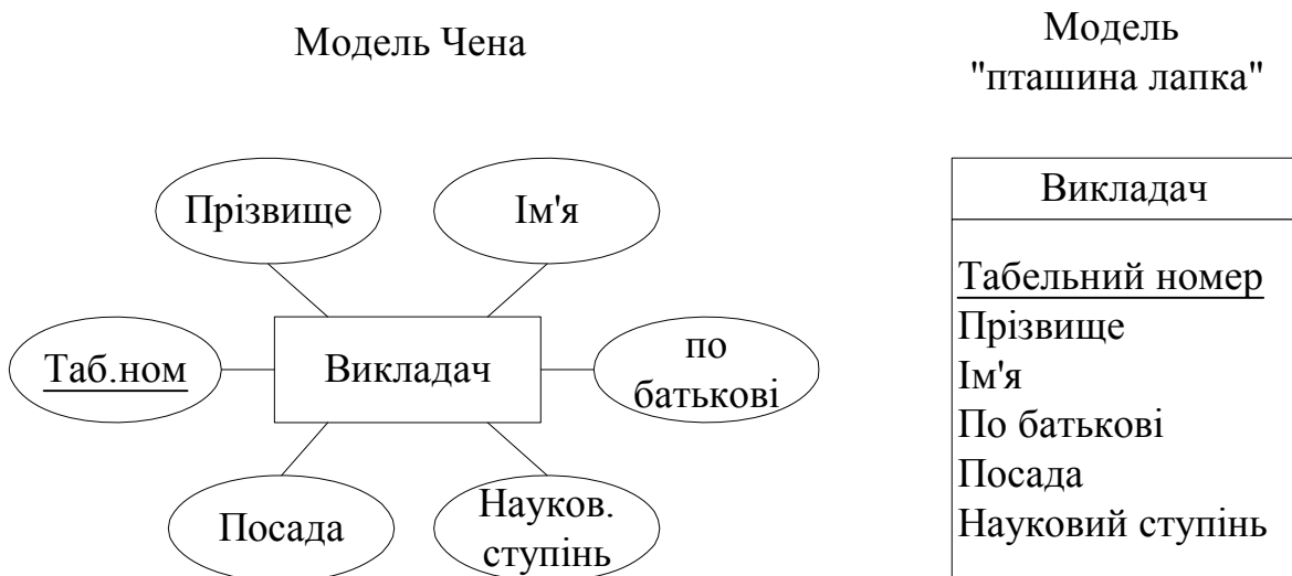
Рис. 5.2. Представлення сутностей і атрибутів у ER-діаграмах П. Чена і ER-діаграмах "пташина лапка"
