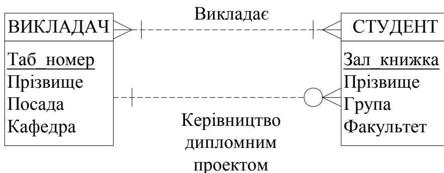
Рис. 5.13. Різні зв'язки між двома сутностями
